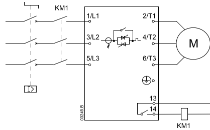
Softstarter mit Überlastschutz und Hauptschutz
