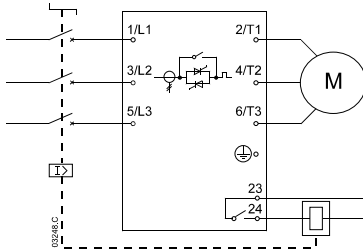
Softstarter mit Überlastschutz
