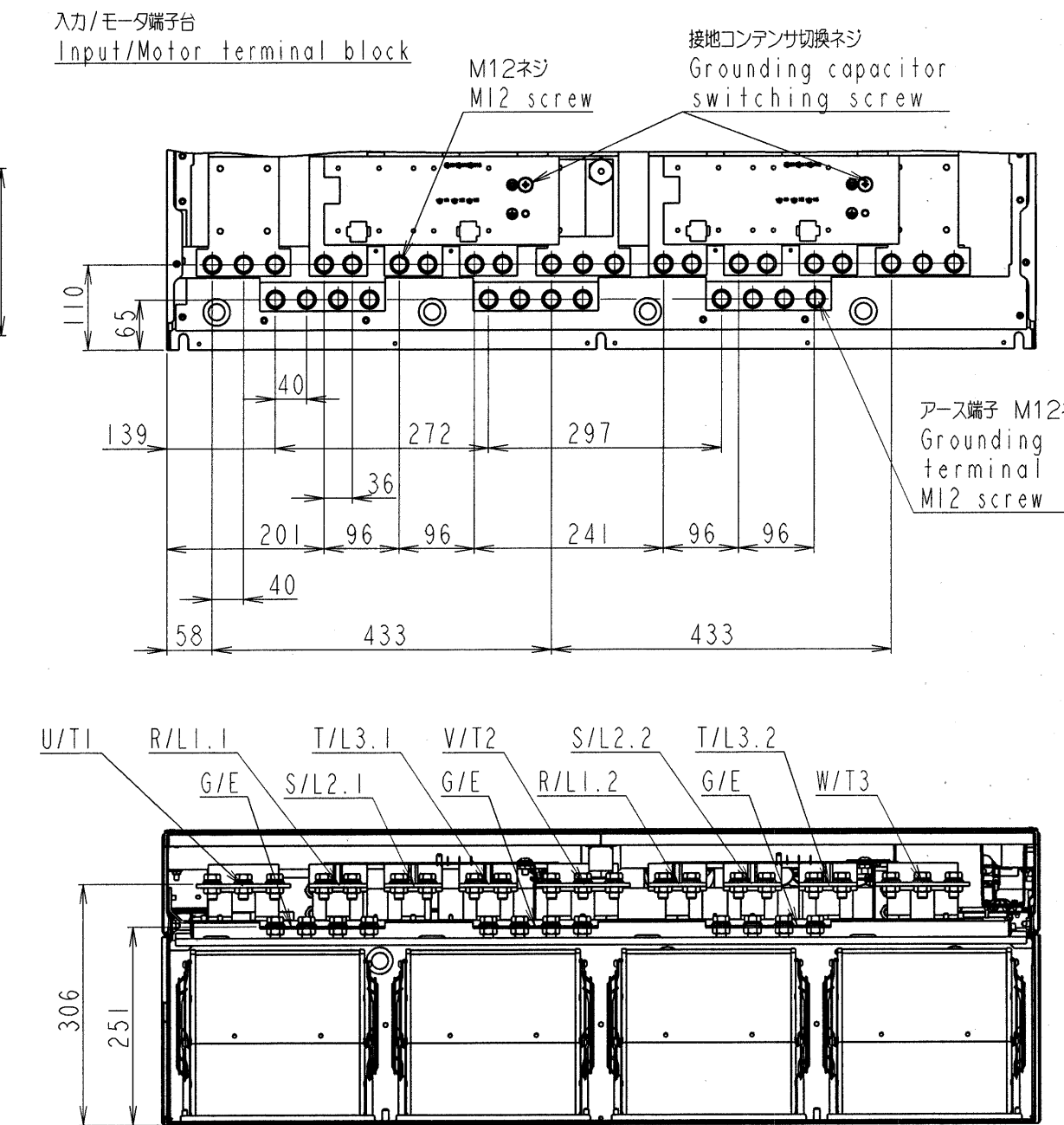
主回路端子台 Main circuit terminal block
