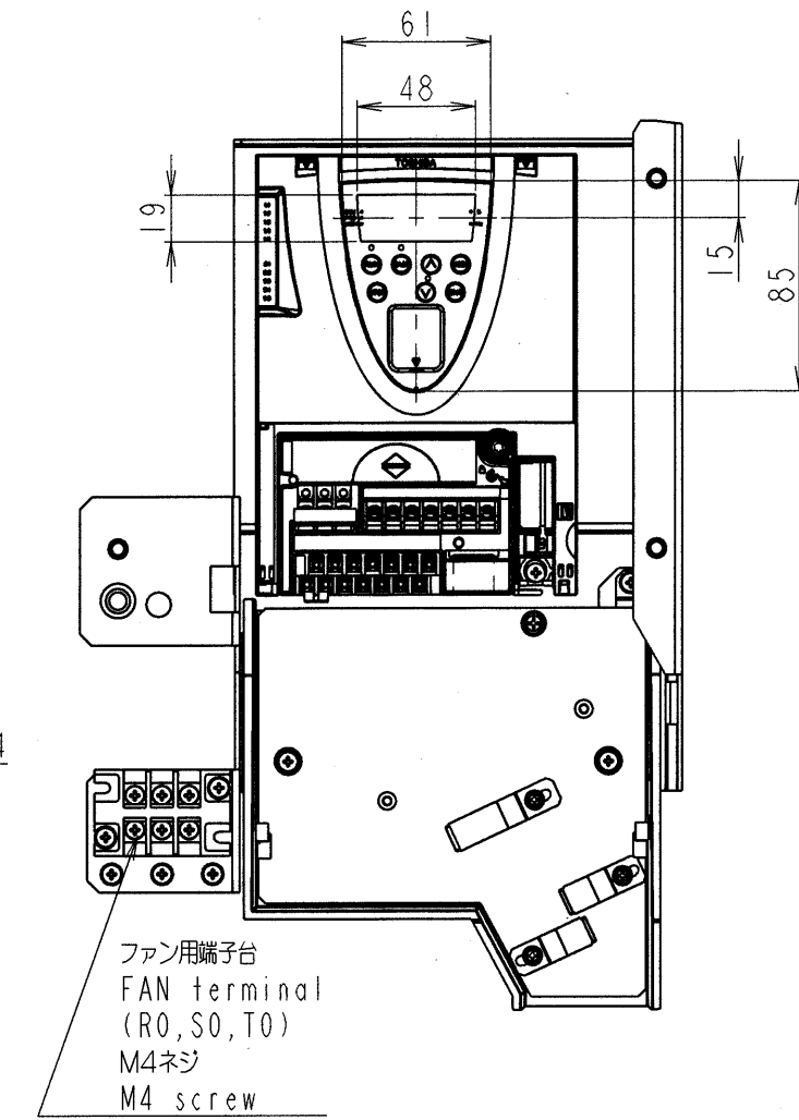
操作パネル Operation panel
