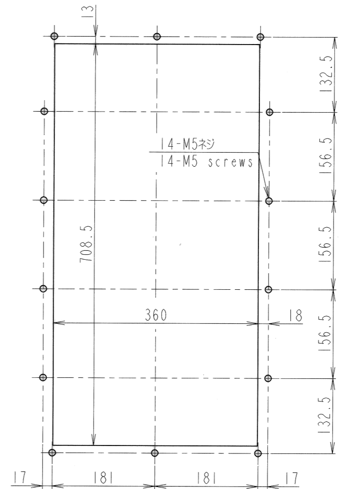
パネルカット寸法 Panel cutout dimension
