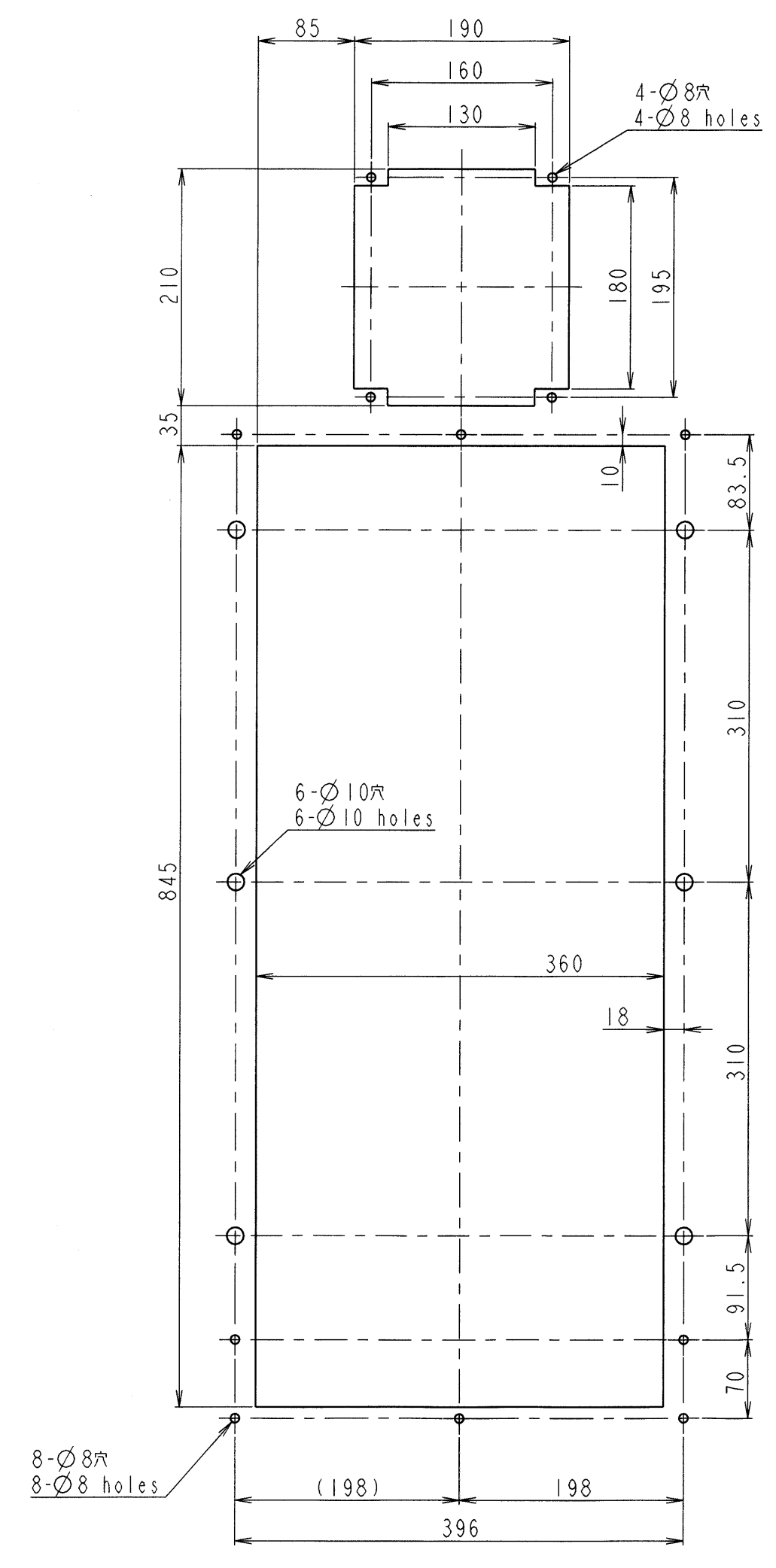
パネルカット寸法 Panel cutout dimension
