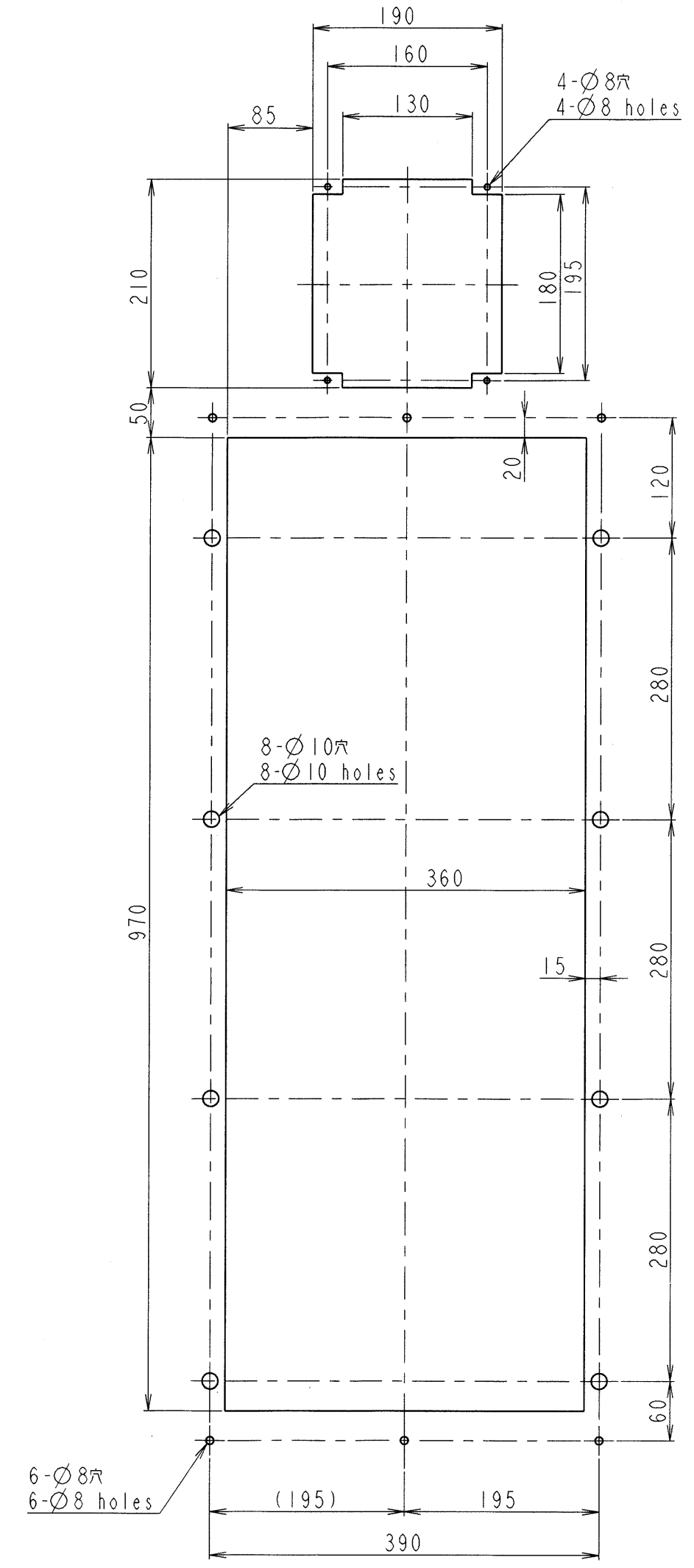
パネルカット寸法 Panel cutout dimension
